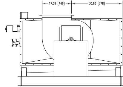
FAN END VIEW
